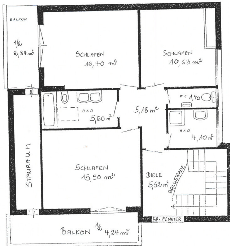
Grundriss OG
