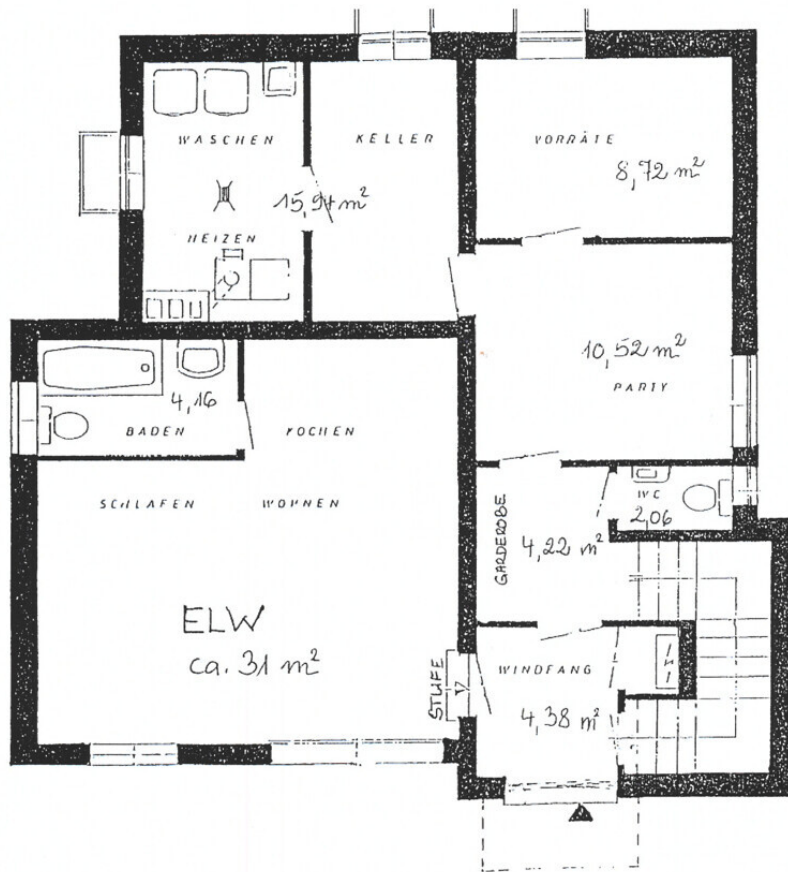
Grundriss UG
