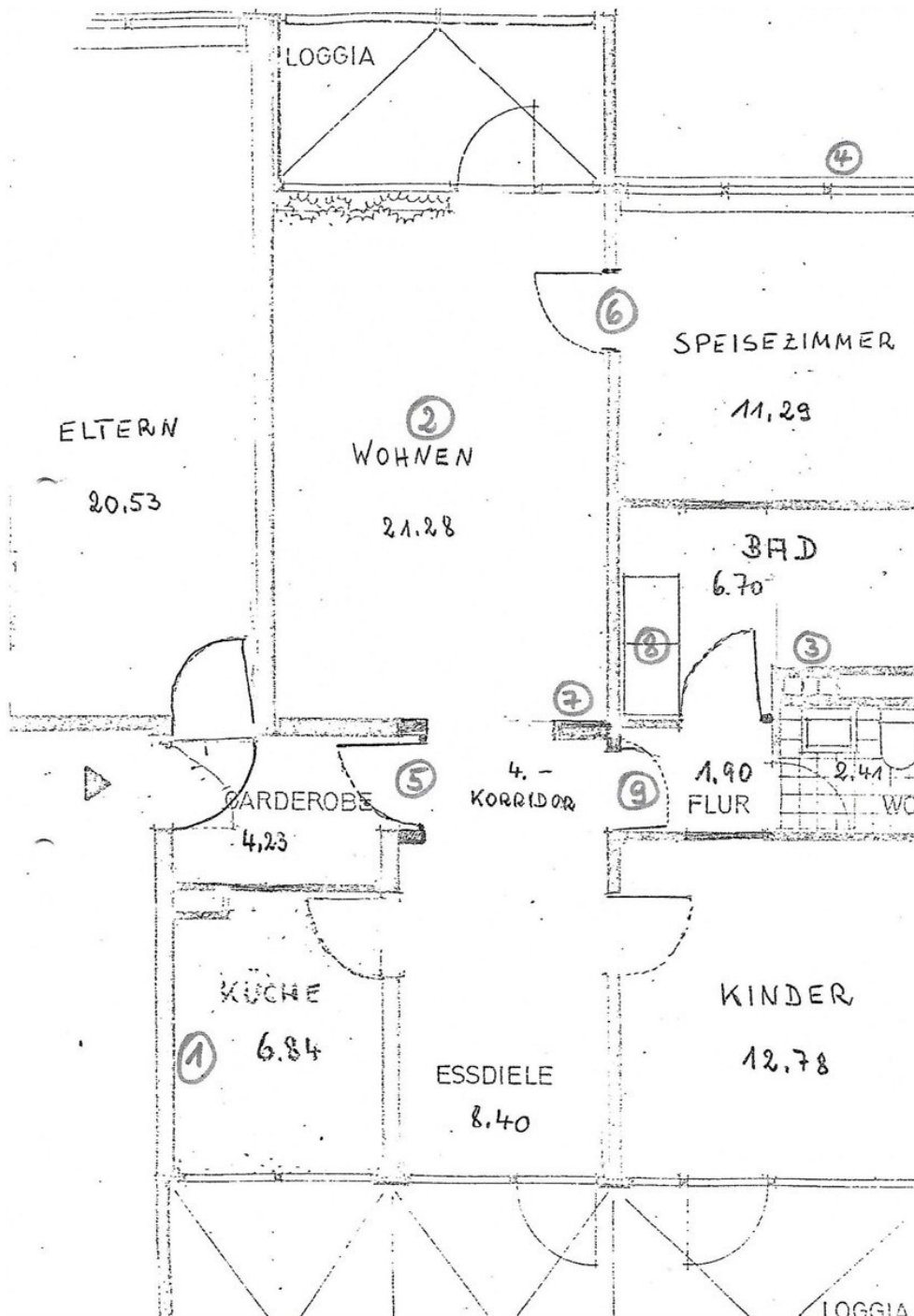
Grundriss
